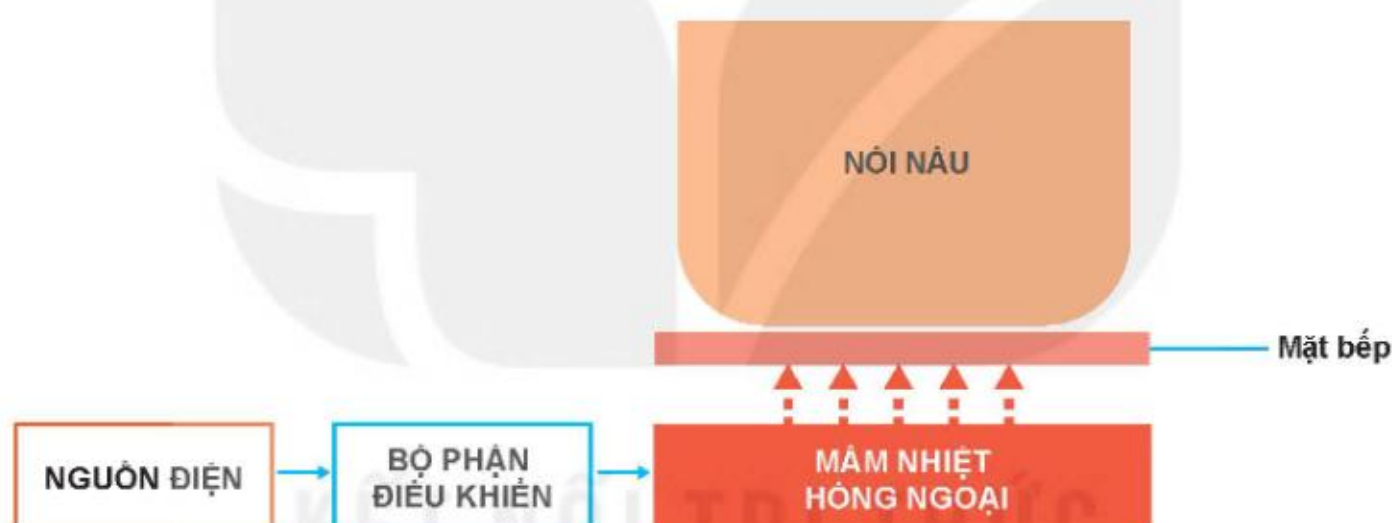
Hình 13.2. Sơ đồ nguyên lí làm việc của bếp hồng ngoại
