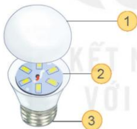
Hình 11.5. Cấu tạo của bóng đèn LED búp
