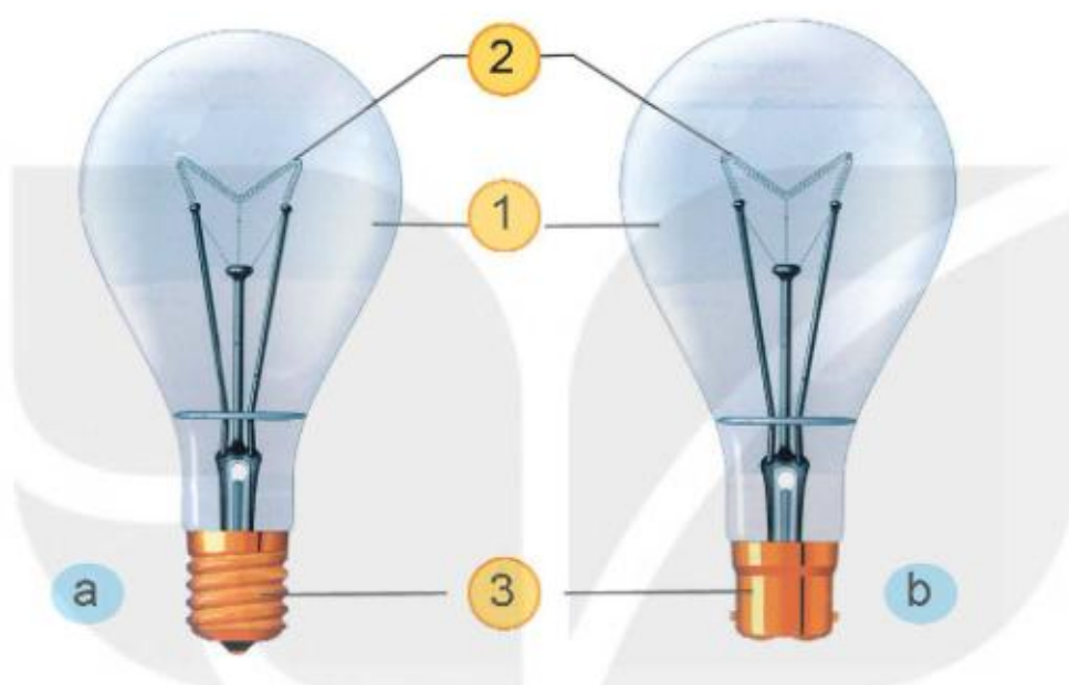
Hình 11.2. Cấu tạo của bóng đèn sợi đốt
