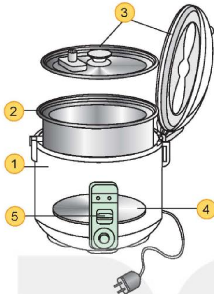
Hình 12.2. Cấu tạo nồi cơm điện
