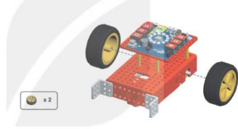
Hình 4.7. Lắp 2 bánh xe
