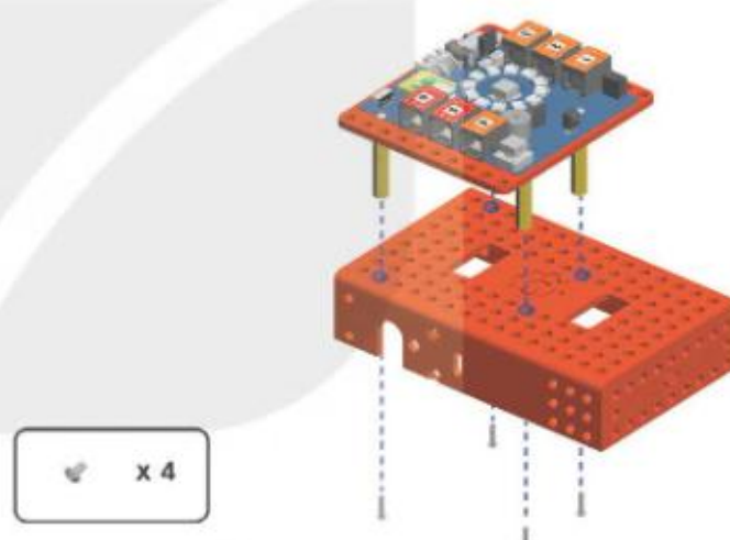
Hình 4.2. Lắp chi tiết ở bước 2 với thân 9 \times 15
