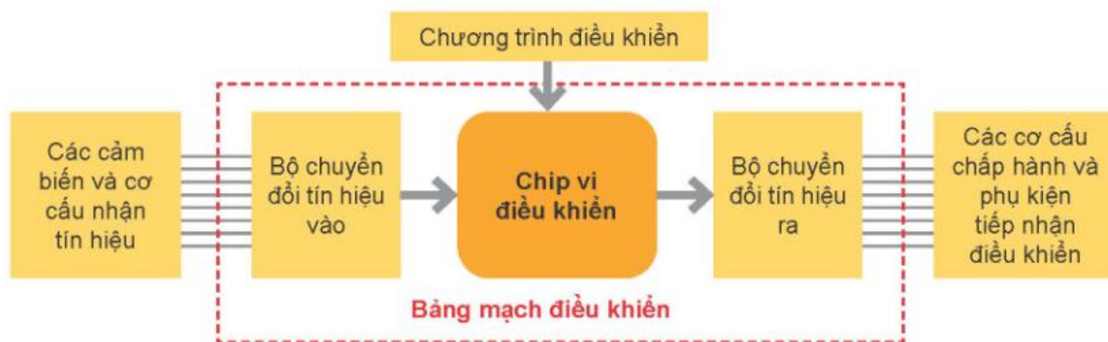
Hình 1.1. Cấu tạo và nguyên lí hoạt động của robot
