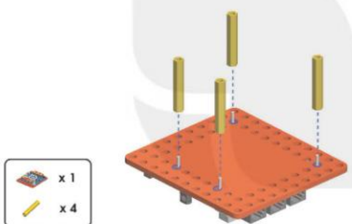
Hình 4.1. Lắp trụ đồng
