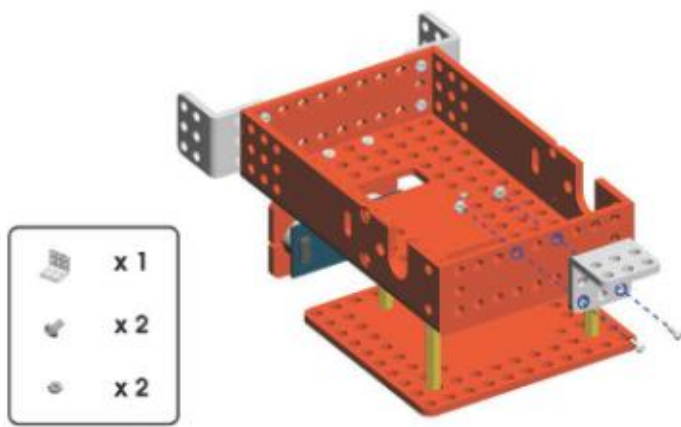
Hình 4.4. Lắp tấm vuông L 2x2x3 vào sau thân 9x15
