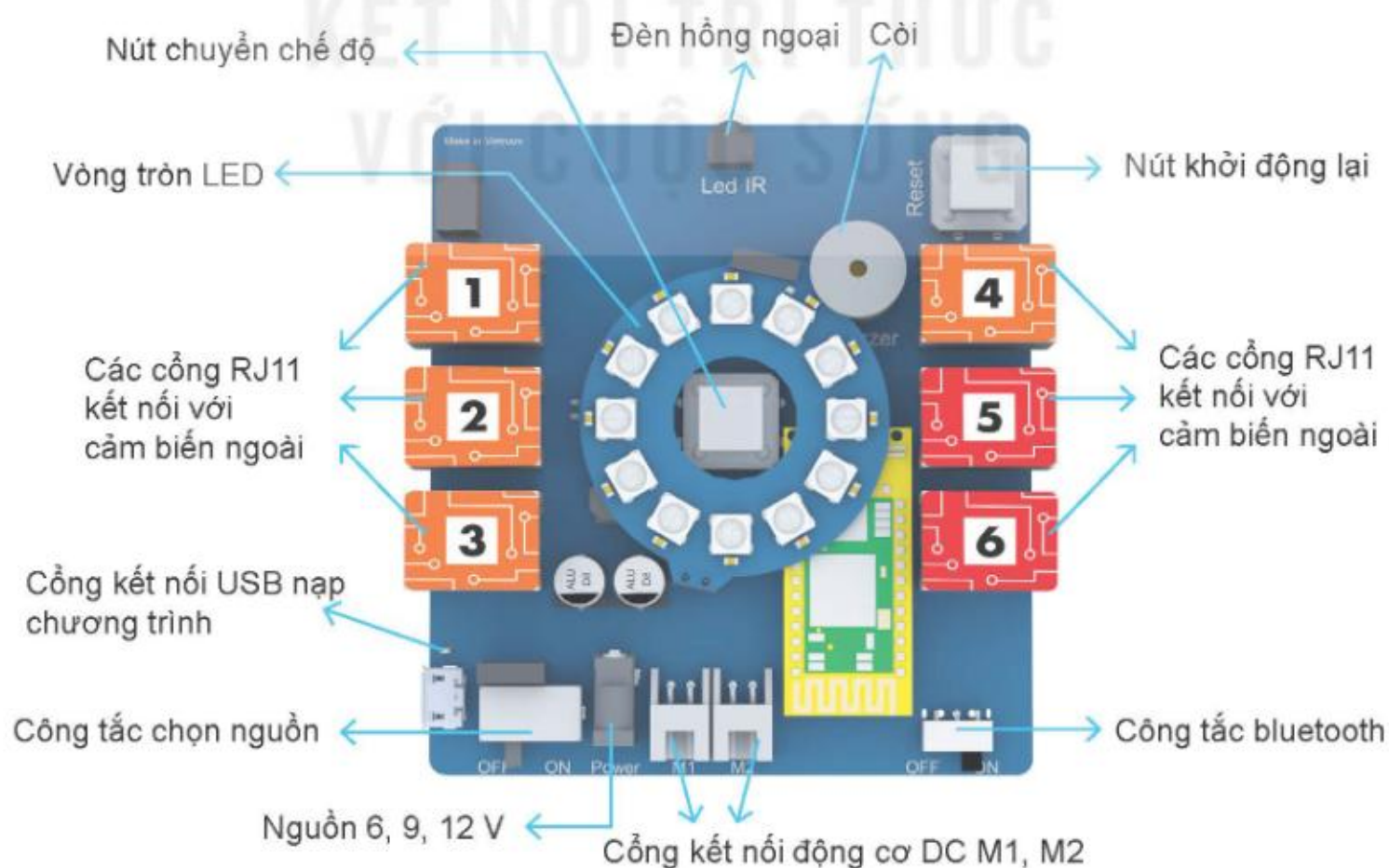
Hình 2.2. Bảng mạch điều khiển của G-Robot
