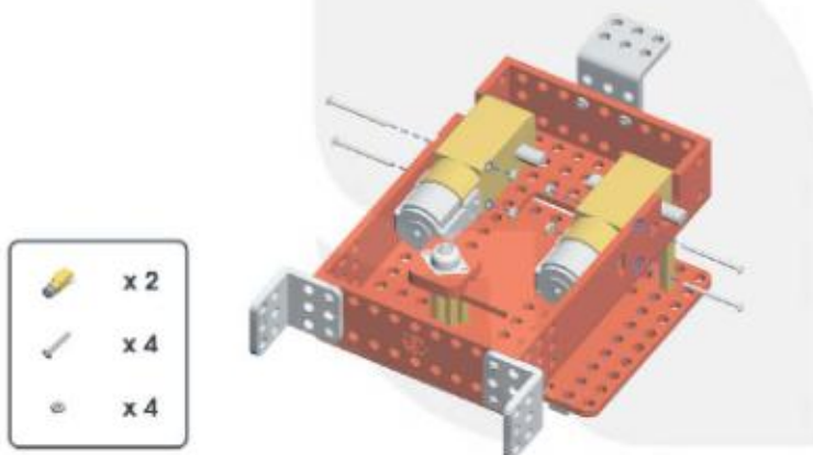
Hình 4.6. Lắp 2 động cơ vào phần dưới thân 9x15
