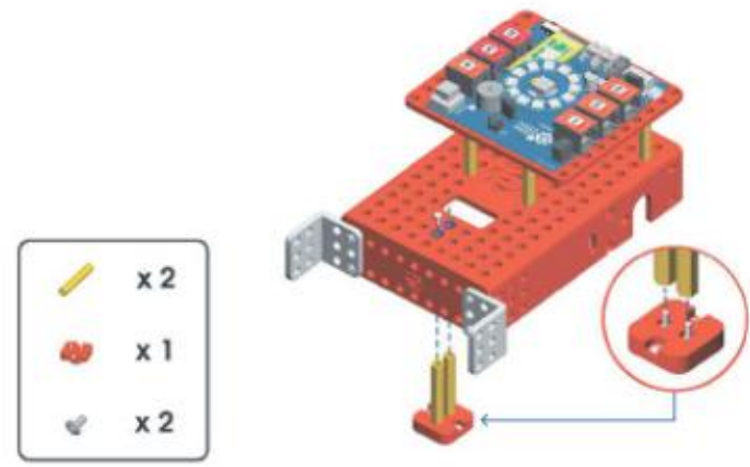
Hình 4.5. Lắp 2 trụ đồng và bánh xe đa hướng vào dưới thân 9x15
