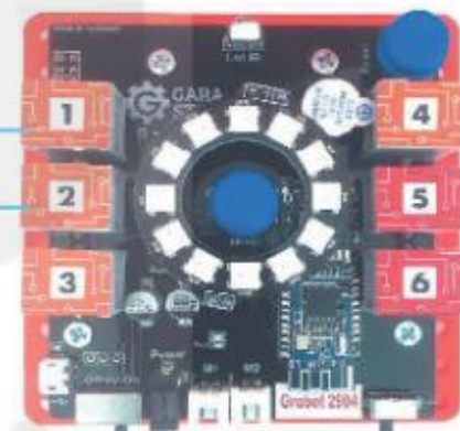
Bảng mạch điều khiển
