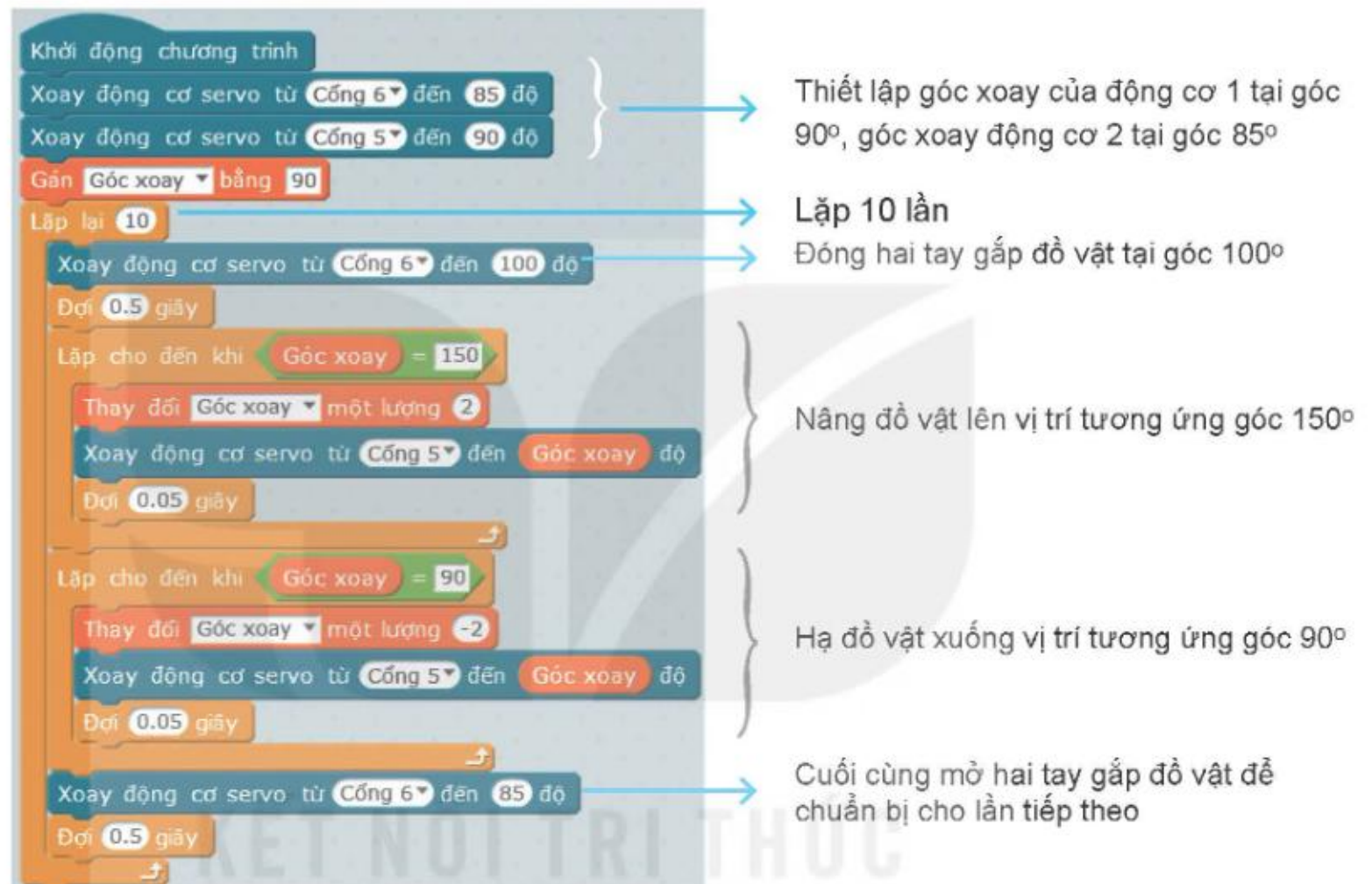
Hình 9.6. Chương trình điều khiển cánh tay hai bậc của robot G-Robot
