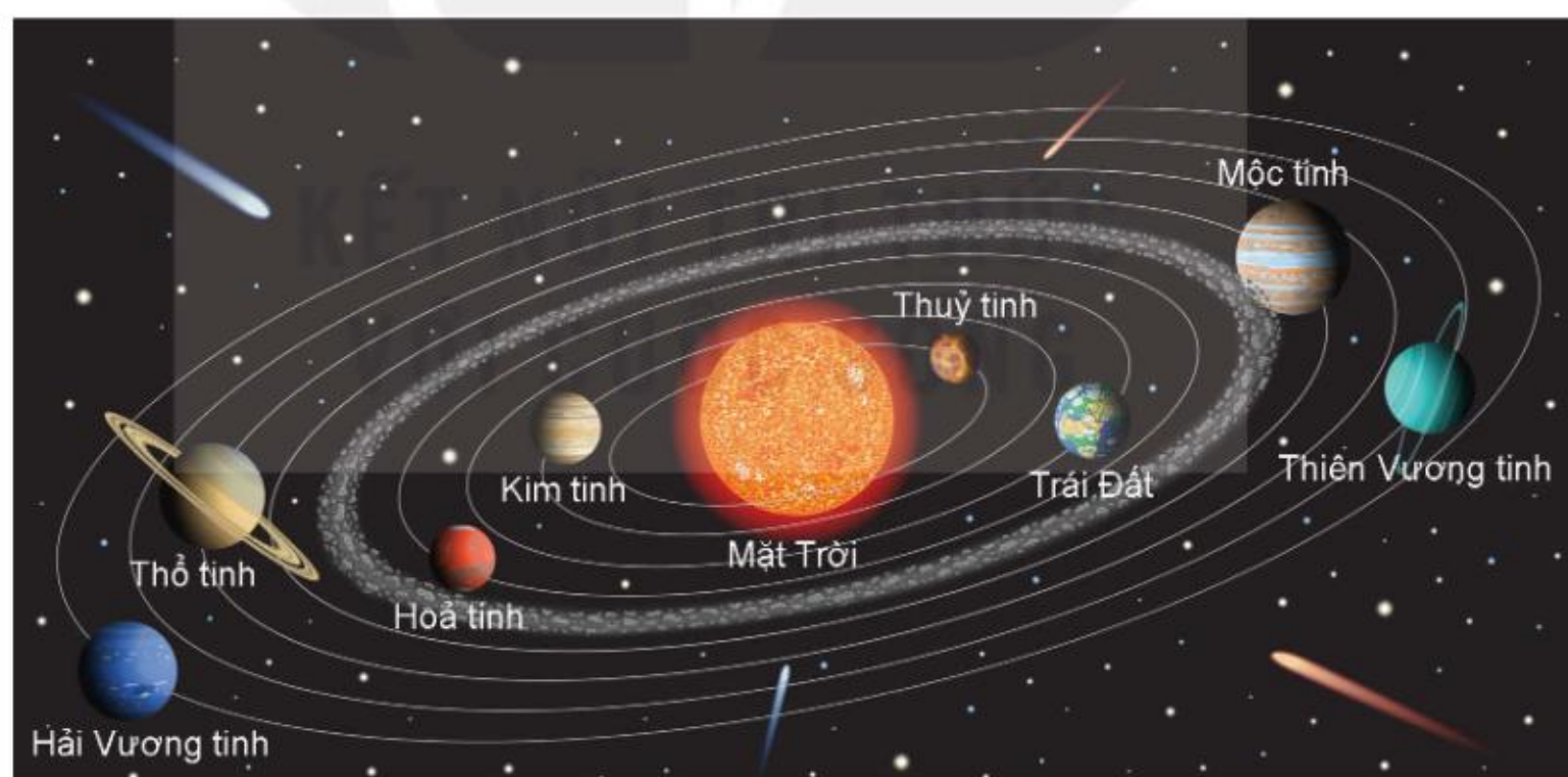
Hình 5.1. Mô hình hệ Mặt Trời
