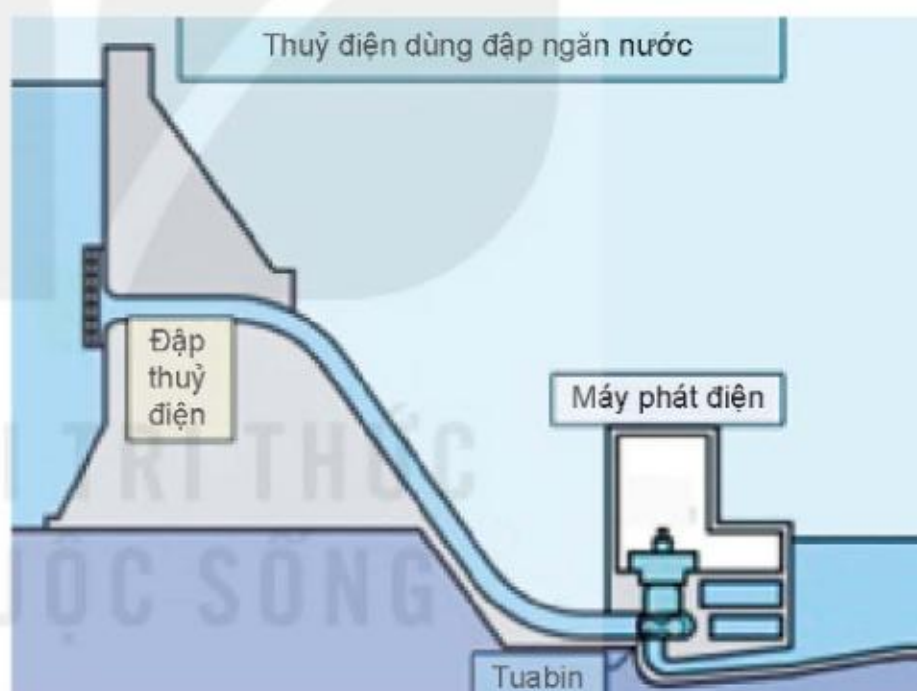
Hình 10.2. Nguyên lí hoạt động nhà máy thủy điện
