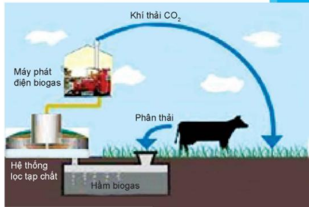
Hình 10.3. Chu trình sản xuất bioga
