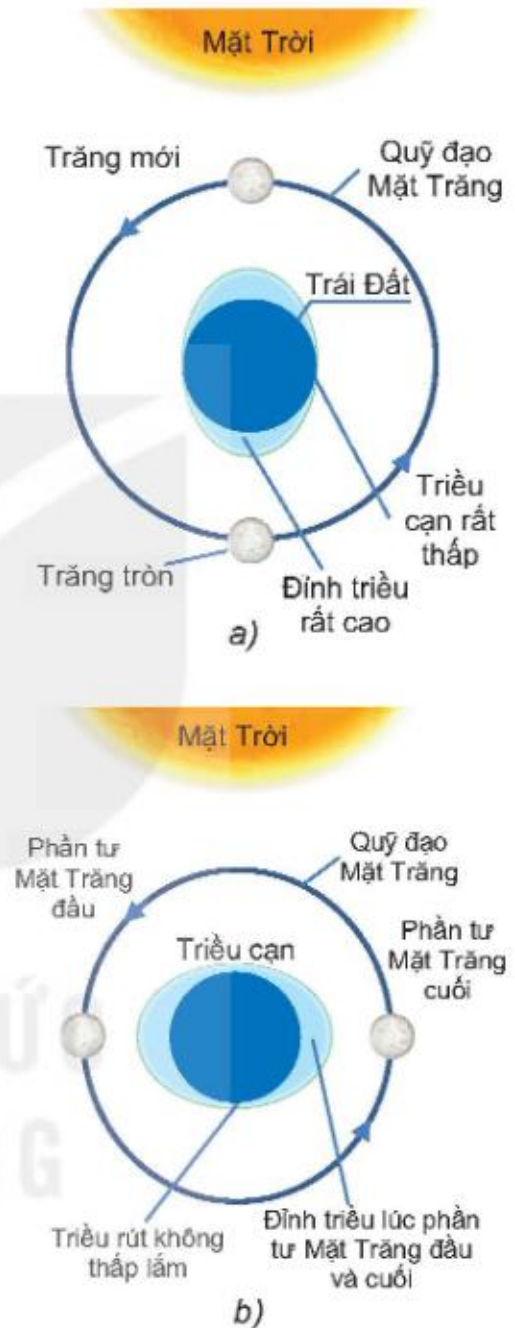
Hình 6.12. Lực hấp dẫn do Mặt Trăng, Mặt Trời tác động lên Trái Đất ở vị trí thẳng hàng (a) và vị trí vuông góc (b)
