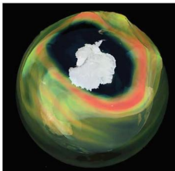
Hình 9.6. Lỗ thủng tầng ozone ở Nam Cực
