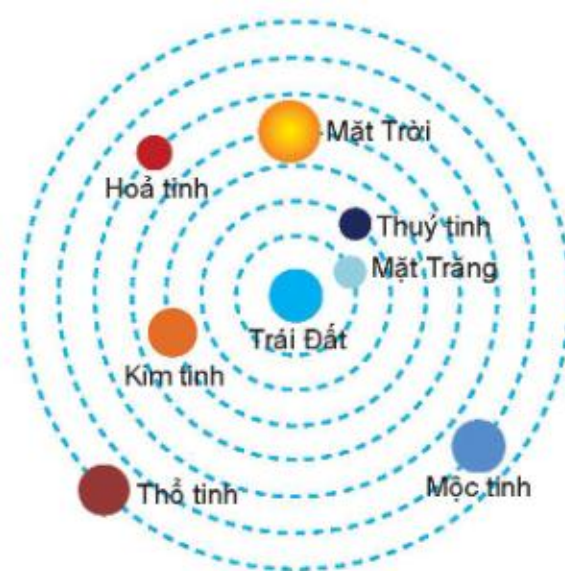
Hình 5.13. Mô hình hệ địa tâm của Ptolemy
