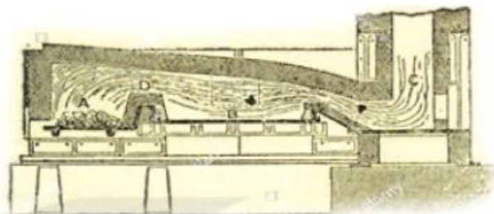
Hình 4. Lò luyện quặng theo phương pháp “pút-đinh” (Hen-ri Côt)
