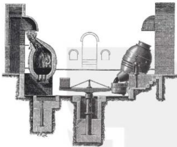
Hình 6. Mô phỏng quá trình luyện thép theo phương pháp lò cao (Hen-ri Bê-sê-mơ, 1856)
