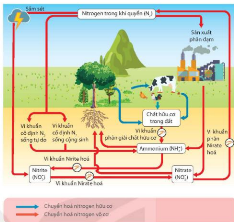
Hình 31.6. Chu trình nitrogen
