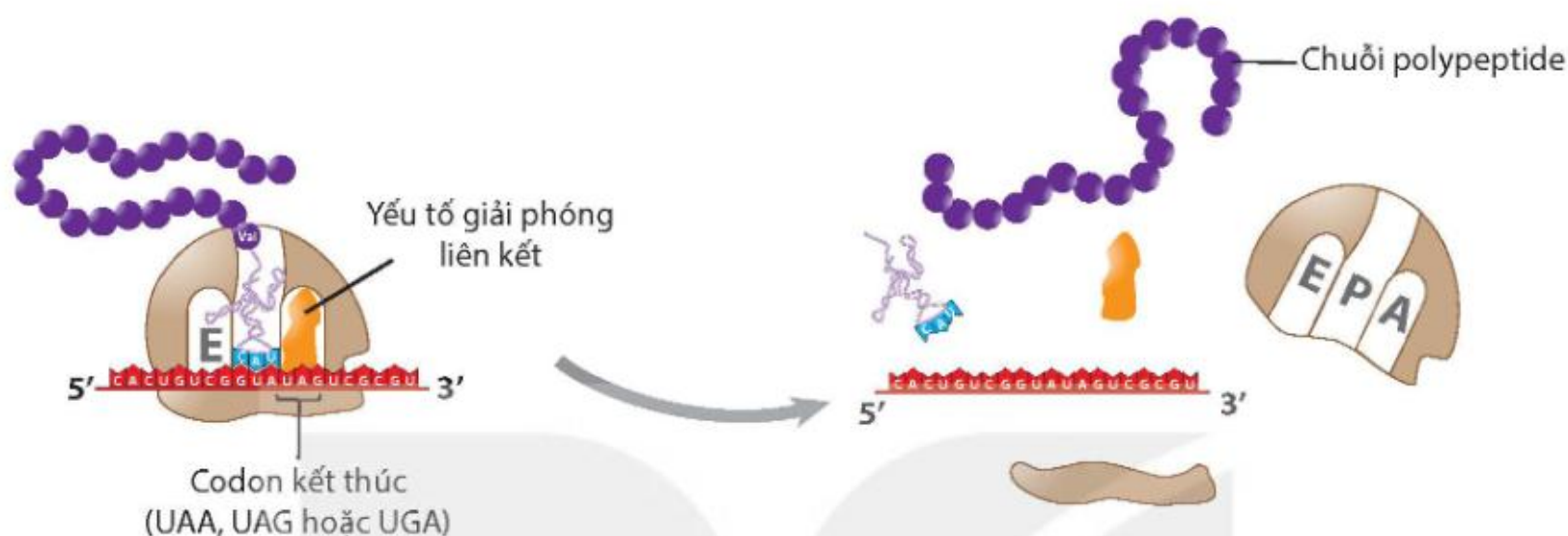
Hình 2.8. Giai đoạn kết thúc dịch mã
