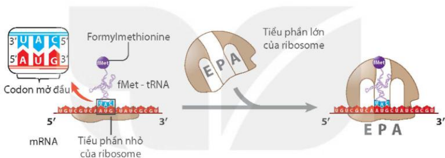
Hình 2.6. Giai đoạn khởi đầu dịch mã
