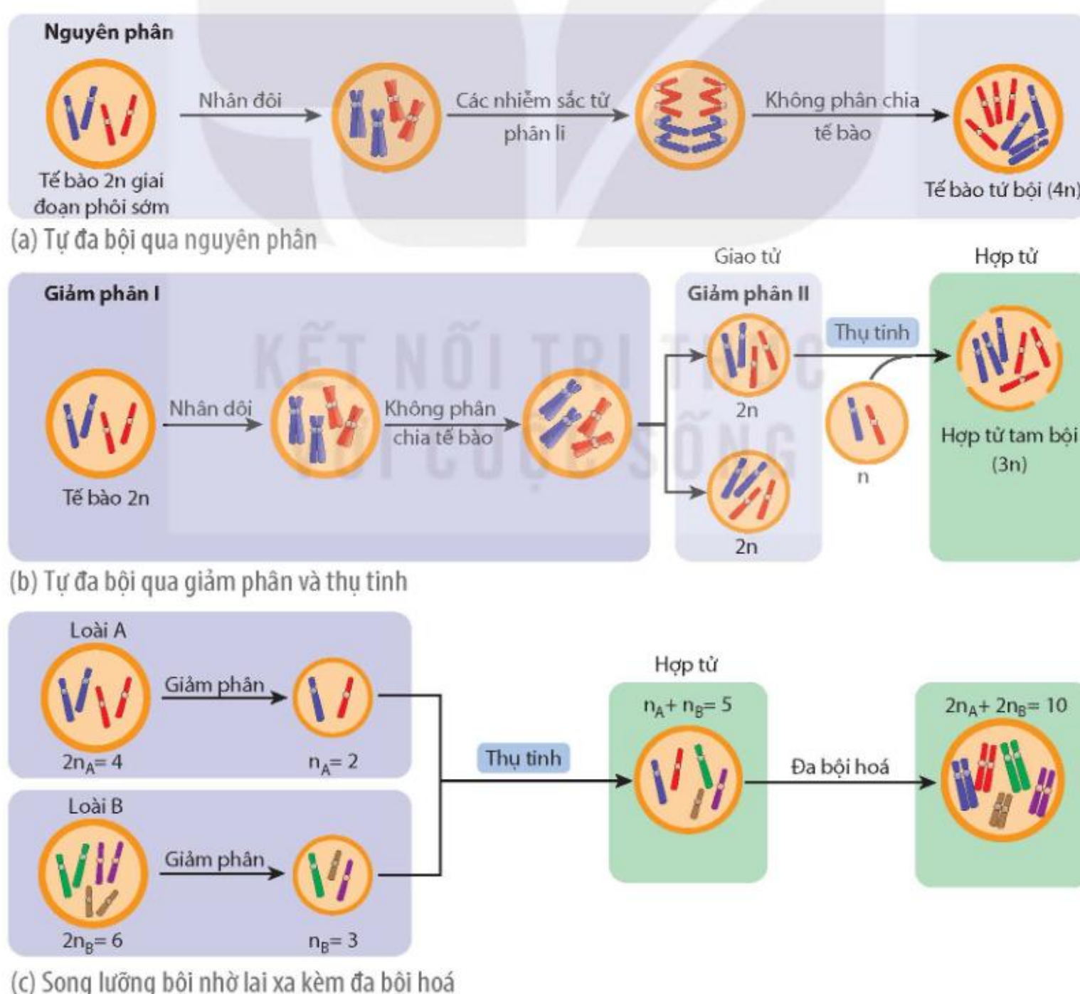
Hình 12.3. Cơ chế phát sinh thể đa bội
