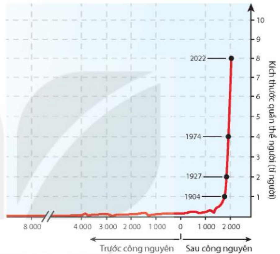
Hình 24.9. Tăng trưởng của quần thể người
