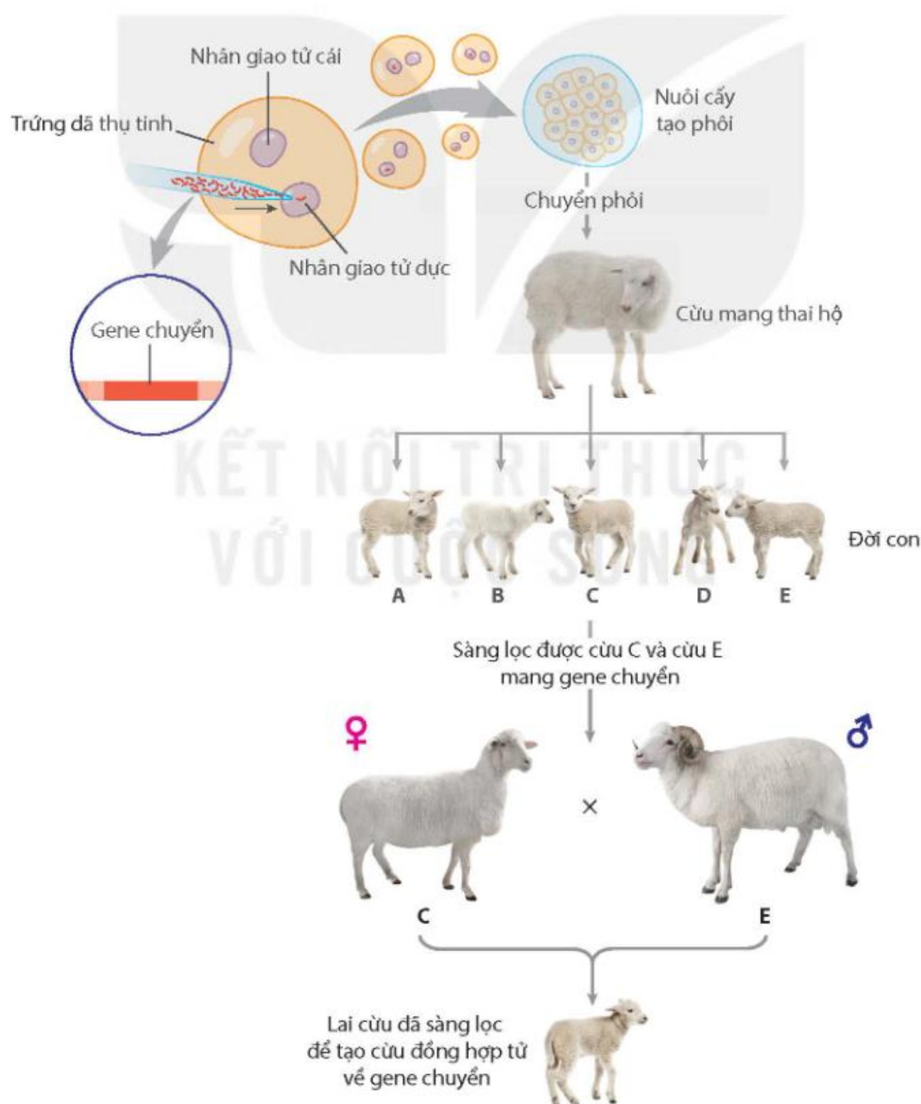
Hình 5.2. Quy trình tạo cừu biến đổi gene
