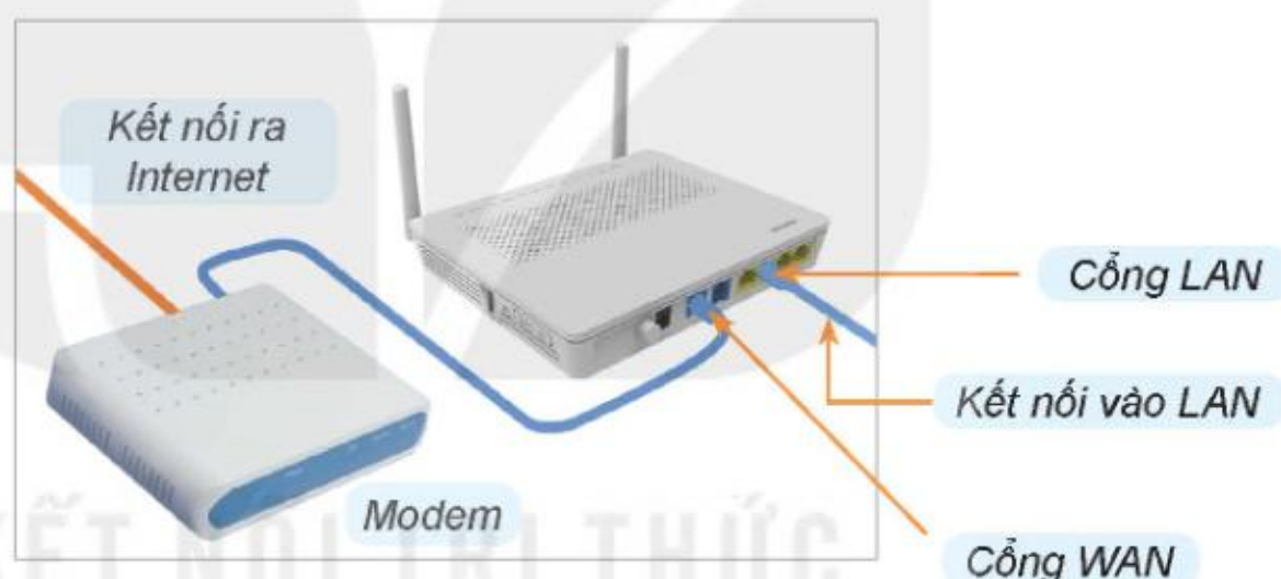
Hình 3.6. Dùng modem kết nối Internet
