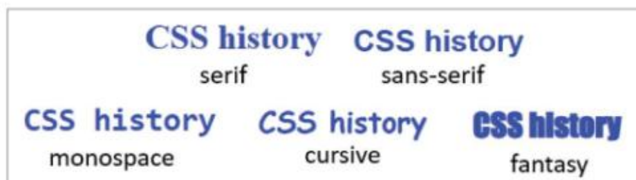
Hình 14.2. Font-family
